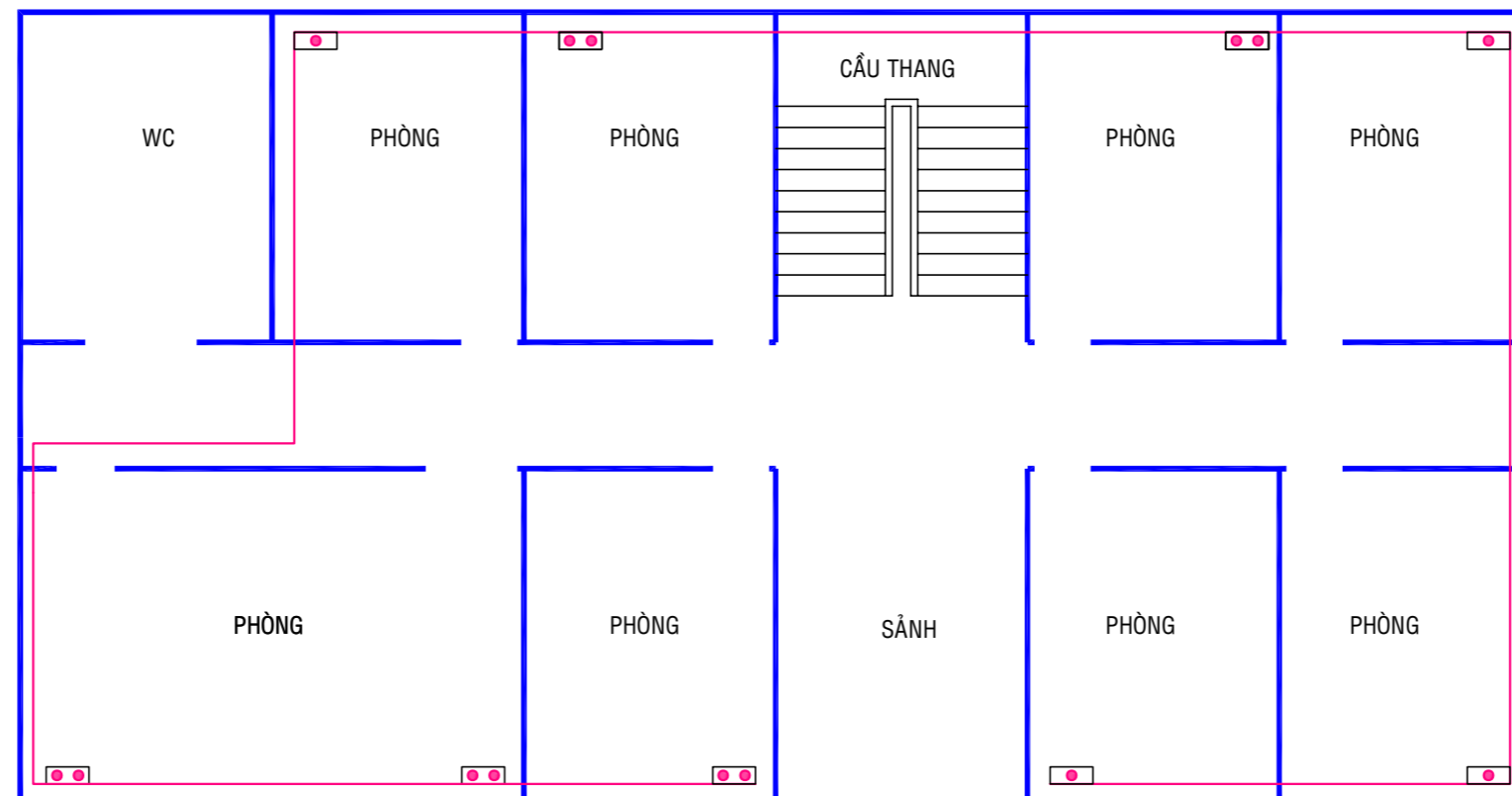
SƠ ĐỒ CẤP MẠNG TẦNG 2
